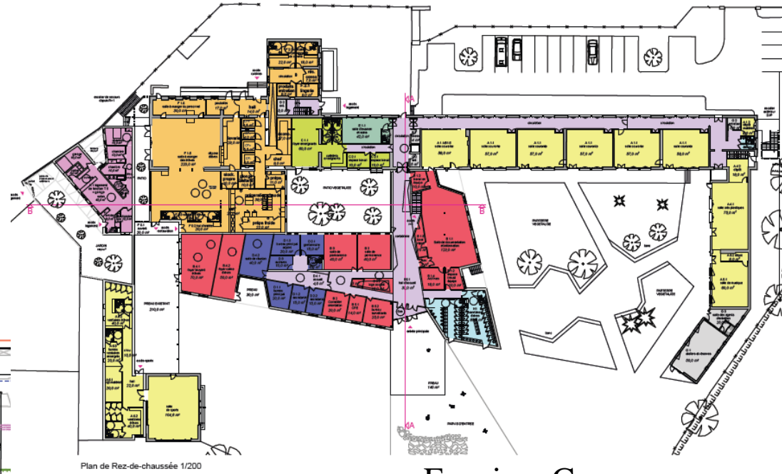
Plan de Rez-de-chaussée 1/200
